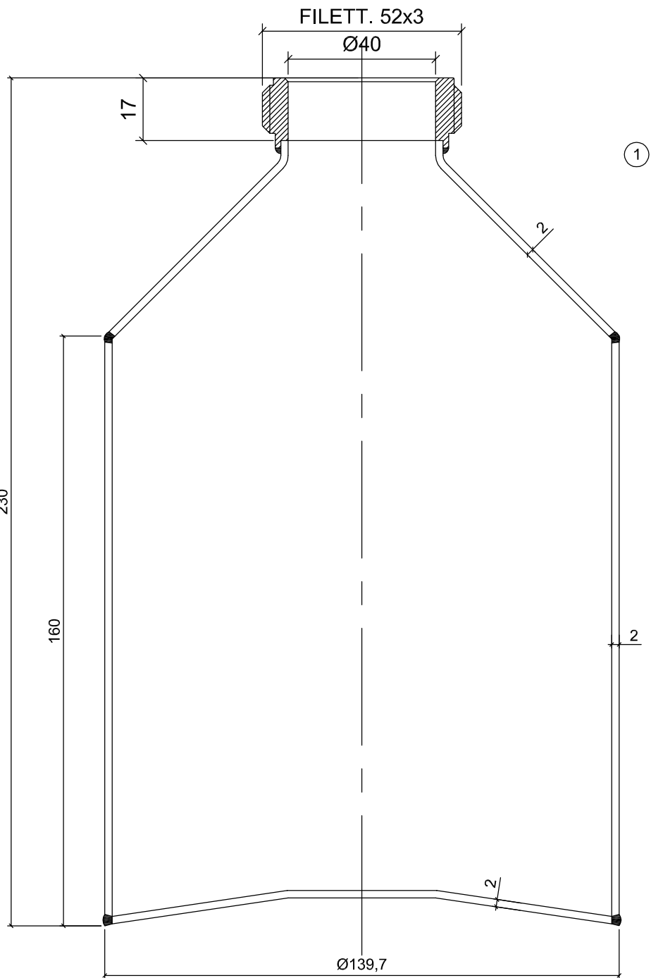
VALVOLA TIPO SO 7420 D6
